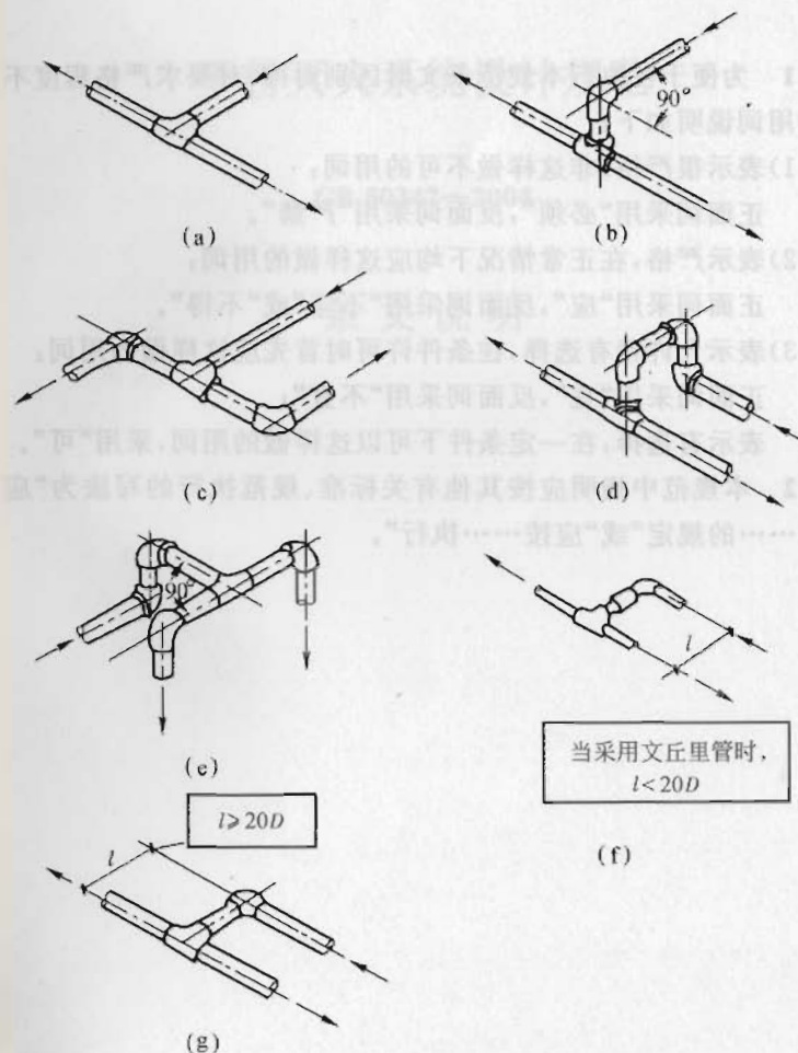
图 B 管网分支结构图
