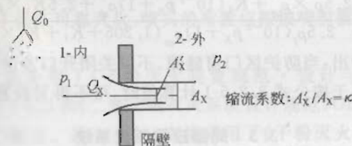
图1 薄壁孔口
